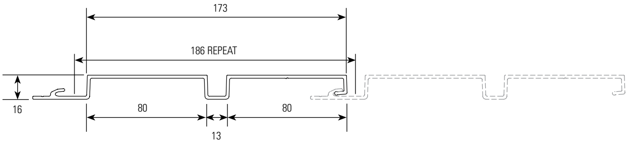
SHADOW 90/90 - SH90/90
