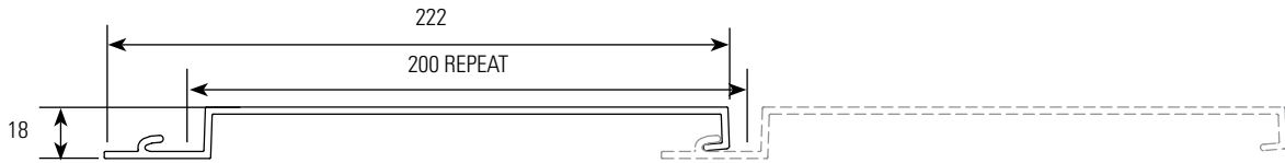
SHADOW 200 - SH200
