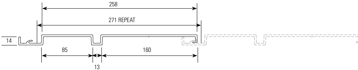
SHADOW 170/95 - SH170/95
